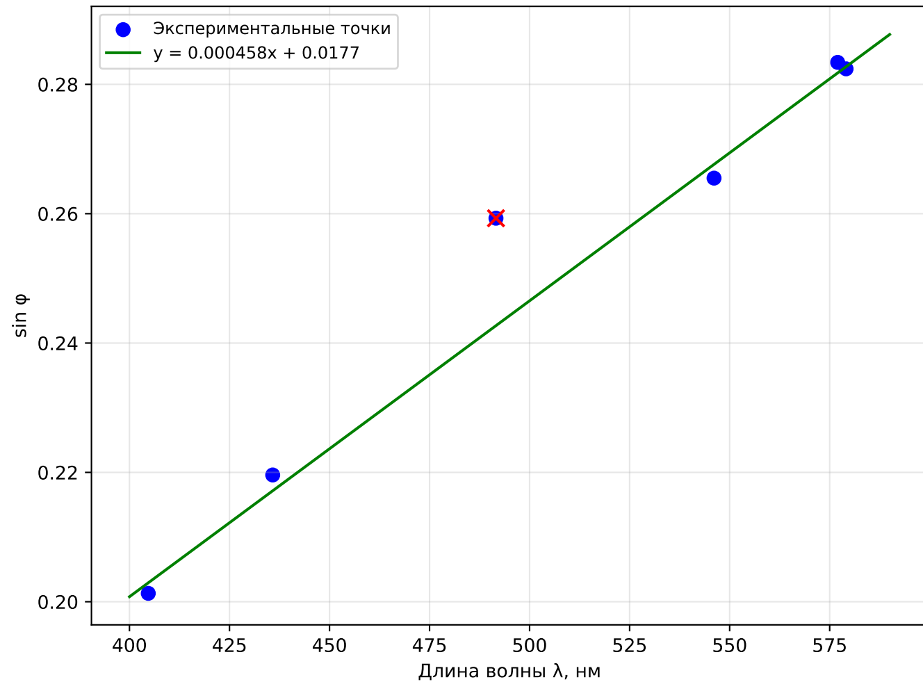
Порядок m = +1
